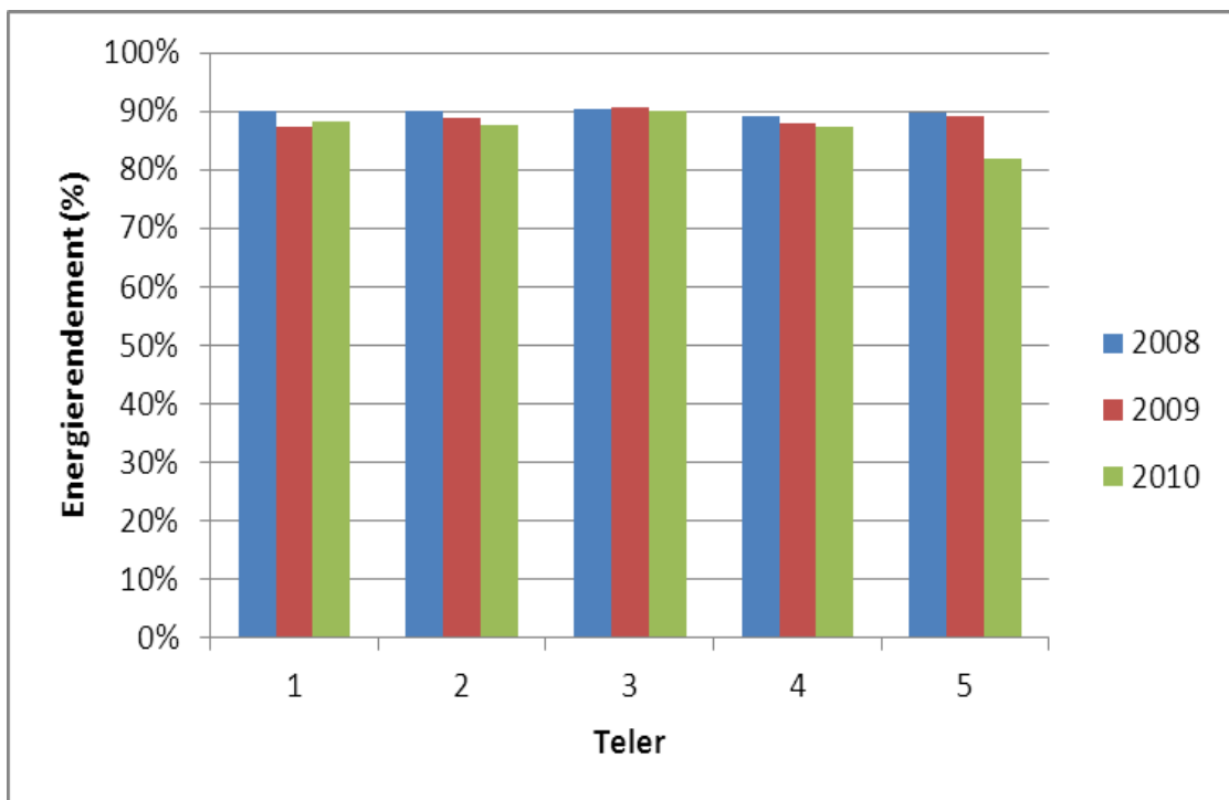
Figuur 3. Energierendement bij vergisting van de hele plant van vijf suikerbietentelers op zandgrond in het project Energieboerderij in de periode 2008-2010. De verschillen tussen telers zijn niet significant.
